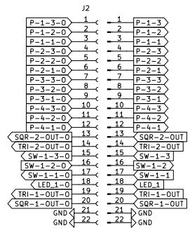
A_Pins_Circuit
