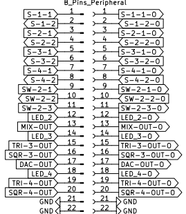
B_Pins_Circuit
